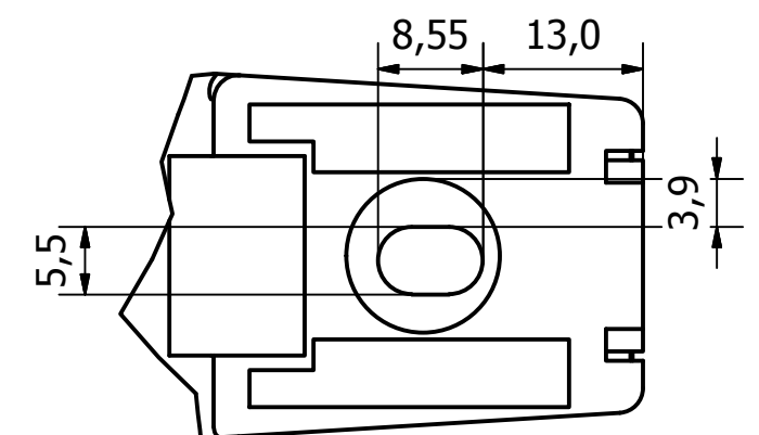
DETAIL A TYP 2 PLACES
